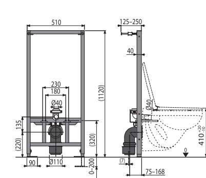
A114/1120 Монтажная рама для подвешного унитаза
