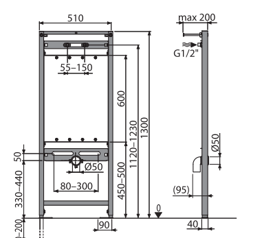
A108/1300 Монтажная рама для мойки и смесителя
