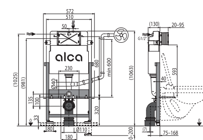
AS101 Sádromodul Скрытая система инсталляции для сухой установки (для гипсокартона)
