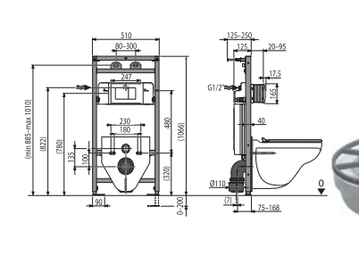
A108F 5:1 SET Сет монтажной рамы, видеюра, изоляционной плиты, откидной решетки и кнопки управления
