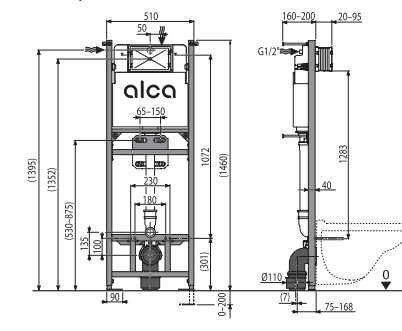
A108F/1500 Монтажная рама с баком для видеюра и смесителя, со стоковым коленом DN90/110
