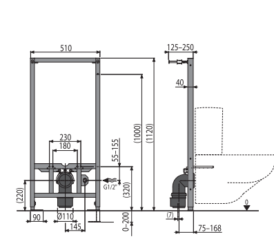
A113/1120 Монтажная рама для подвешного унитаза компакт
