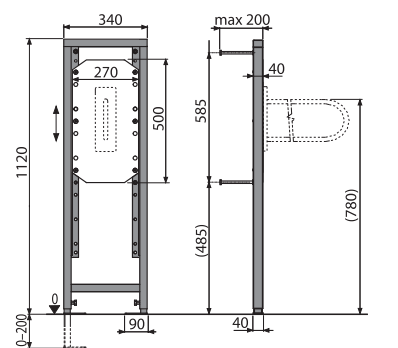
A106/1120 Монтажная рама для поручней
