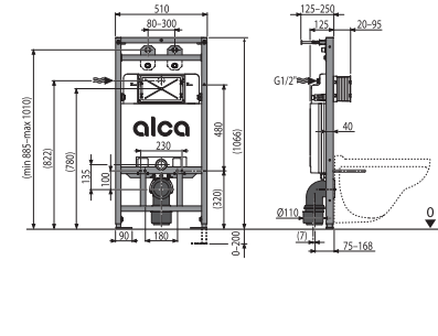
A108F/1100 Монтажная рама с баком для видеюра и смесителя, со стоковым коленом DN90/110
