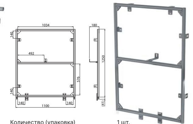
AS101-SET02, AS101-SET02-PR * Системная стена
