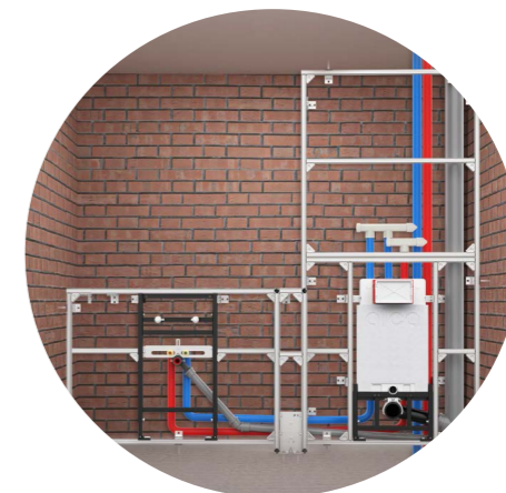
Стенка системы Alcasystem
